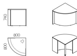
Comptoir d'angle bas, courbe h : 740 mm
