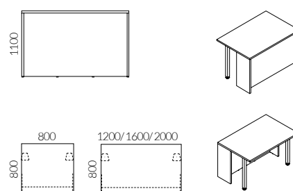
Comptoir droit bas h : 740 mm
