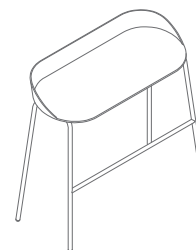
TE02HF 1020 / 430 / 934 11 kg
