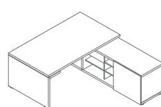
MIT1P 2000-2278 / 2080 / 740 230.05 kg
