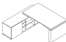
MITF28RL 1990 / 2080 / 1300-760 426.6 kg
