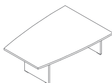
MIT06 2000 / 1000-1400 / 740 154.15 kg
