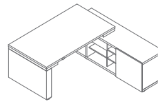
MIT2RP 1990 / 2080 / 1300-760 348.3 kg
