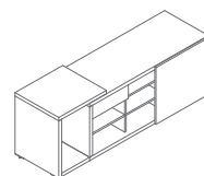
MIT5 1887 / 572 / 690 141.5 kg
