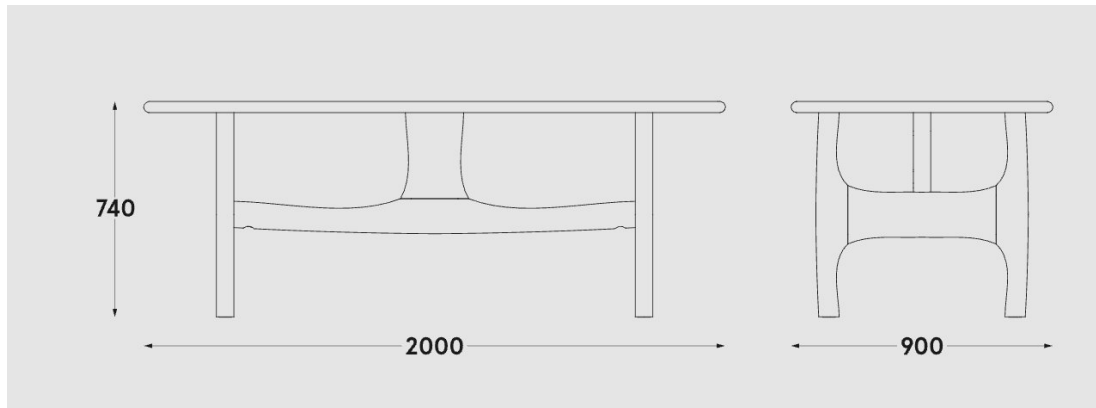
Vue de face et vue de profil — cotes exprimées en millimètres (mm)
