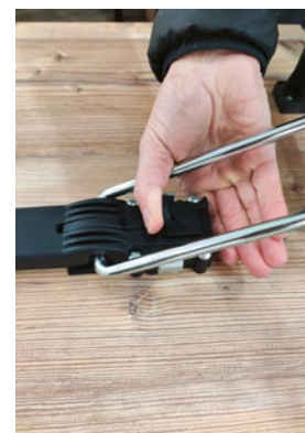
Poignées de déblocage des piétements sous les plateaux
