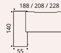
Bureau individuel sur console B-box vue de dessus
