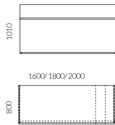
Comptoir Axer type U
