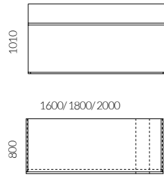
Comptoir Axer typ L
